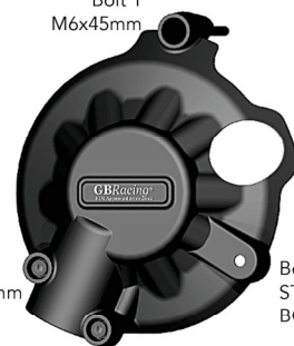
Bolt 3 M6x20mm + M6 Washer
