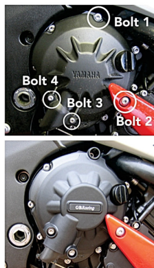
Bolt 4 M6x20mm + M6 Washer
